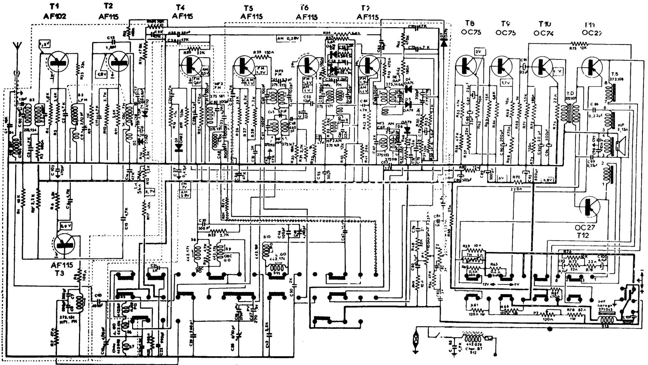
Schema elettrico del radiorecettore SINUDYNE Mod. 3700 Radiomatic
